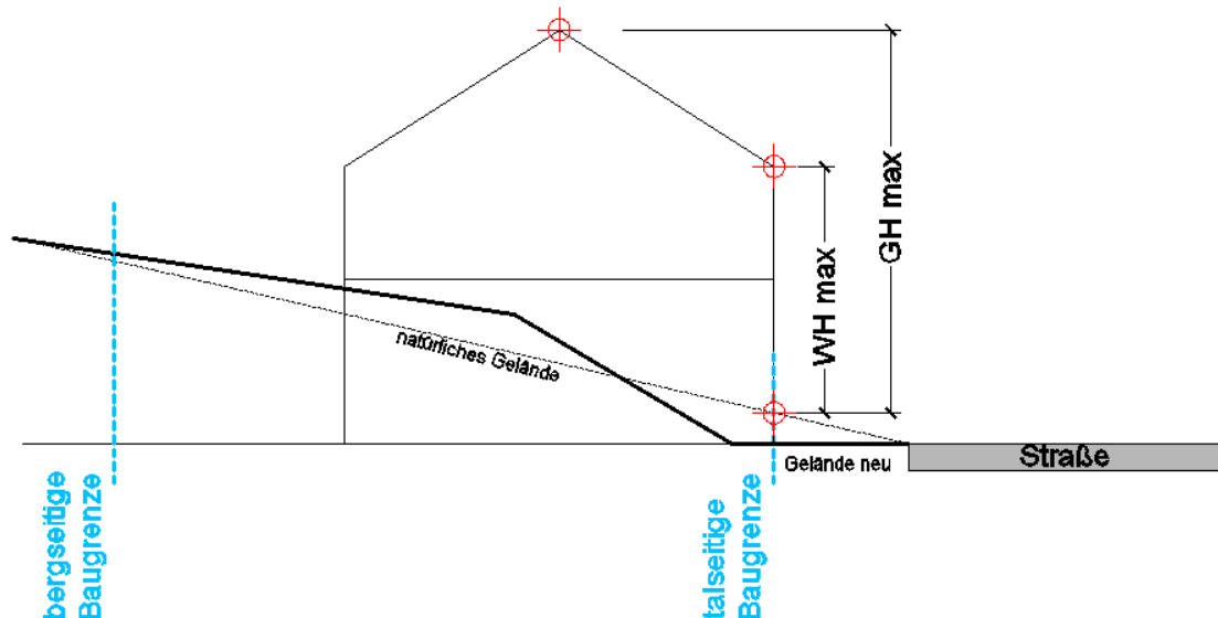
Abbildung 1: Erläuterungsskizze für BQ 1-4, zweiseitig geneigtes Dach (Walmdach)
